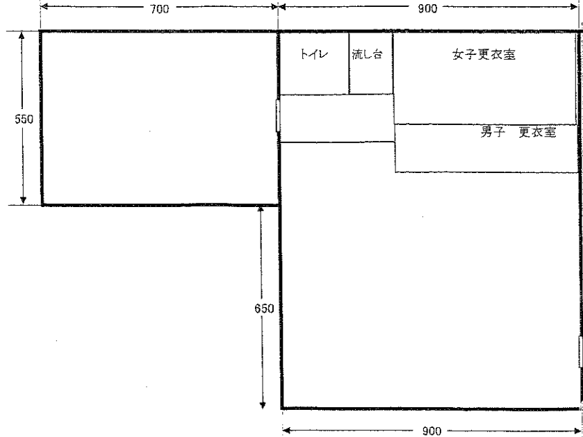
【2F平面図】
