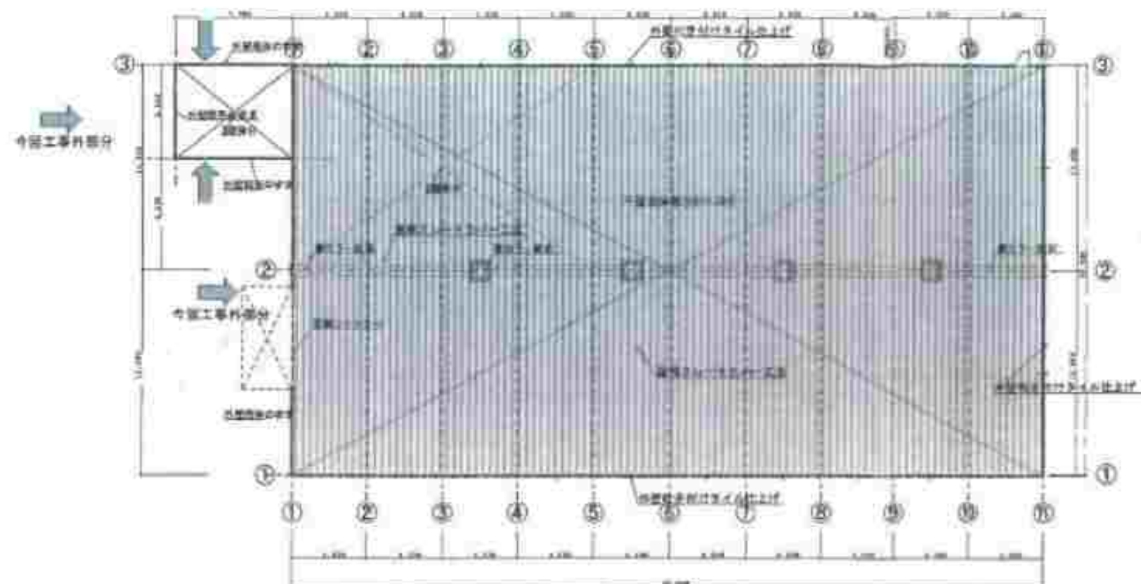
平面図 1/200
