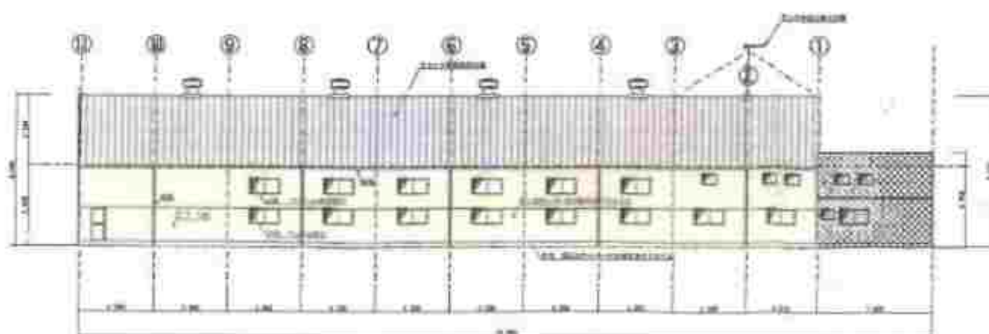
東立面図 1/200
