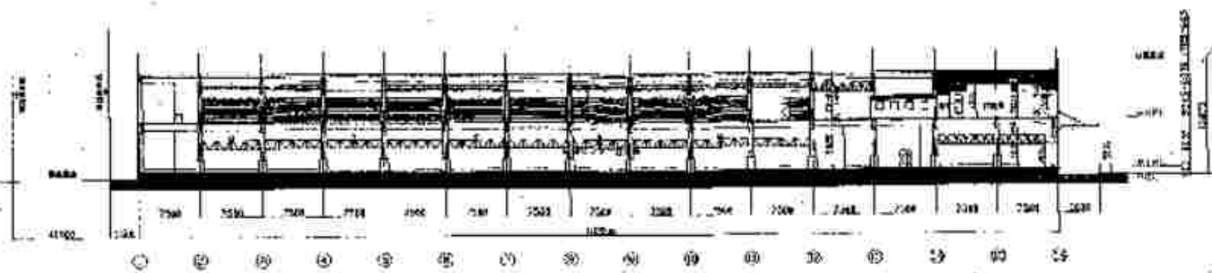
断面図 (1) - (14)
